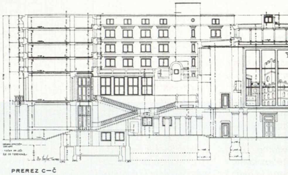
PREREZ C-Č
